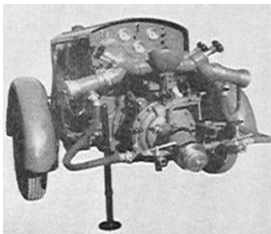
Svensk påhængssprøjet (type API 120). Fra Gysinge Brandcenter.
